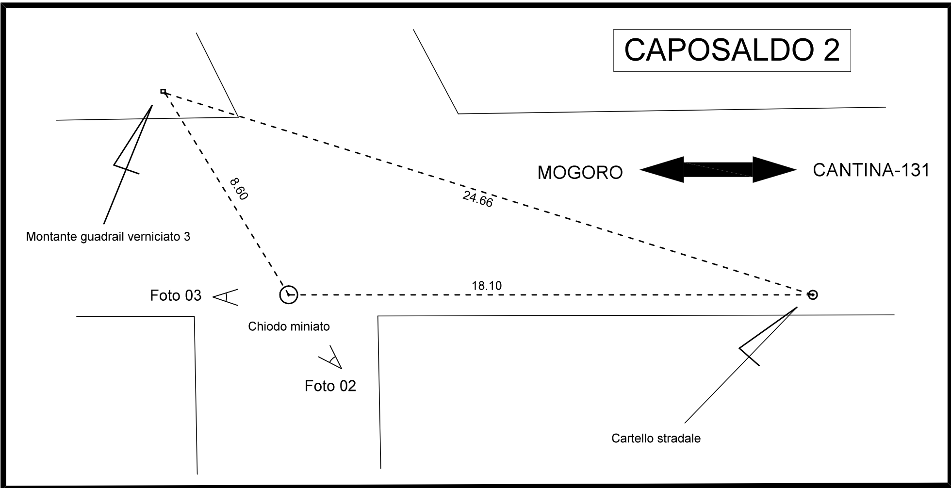
CAPOSALDO N.2: CHIODO AL BORDO DELLA VECCHIA STRADA PROVINCIALE DISMESSA
