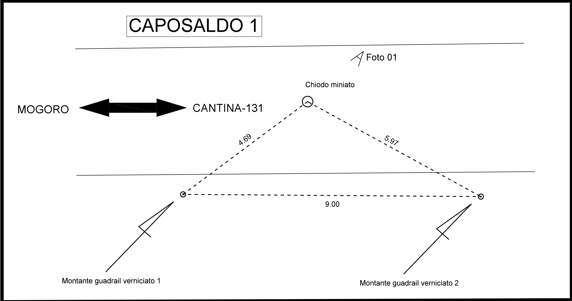
CAPOSALDO N.1: CHIODO IN ASSE LUNGO LA VECCHIA STRADA PROVINCIALE DISMESSA
